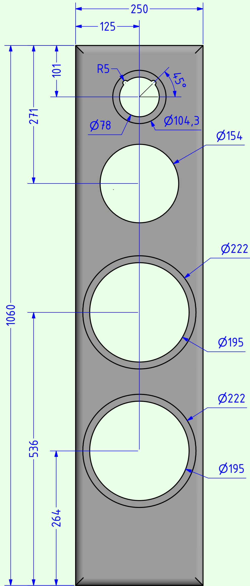
äußere Schallwand
