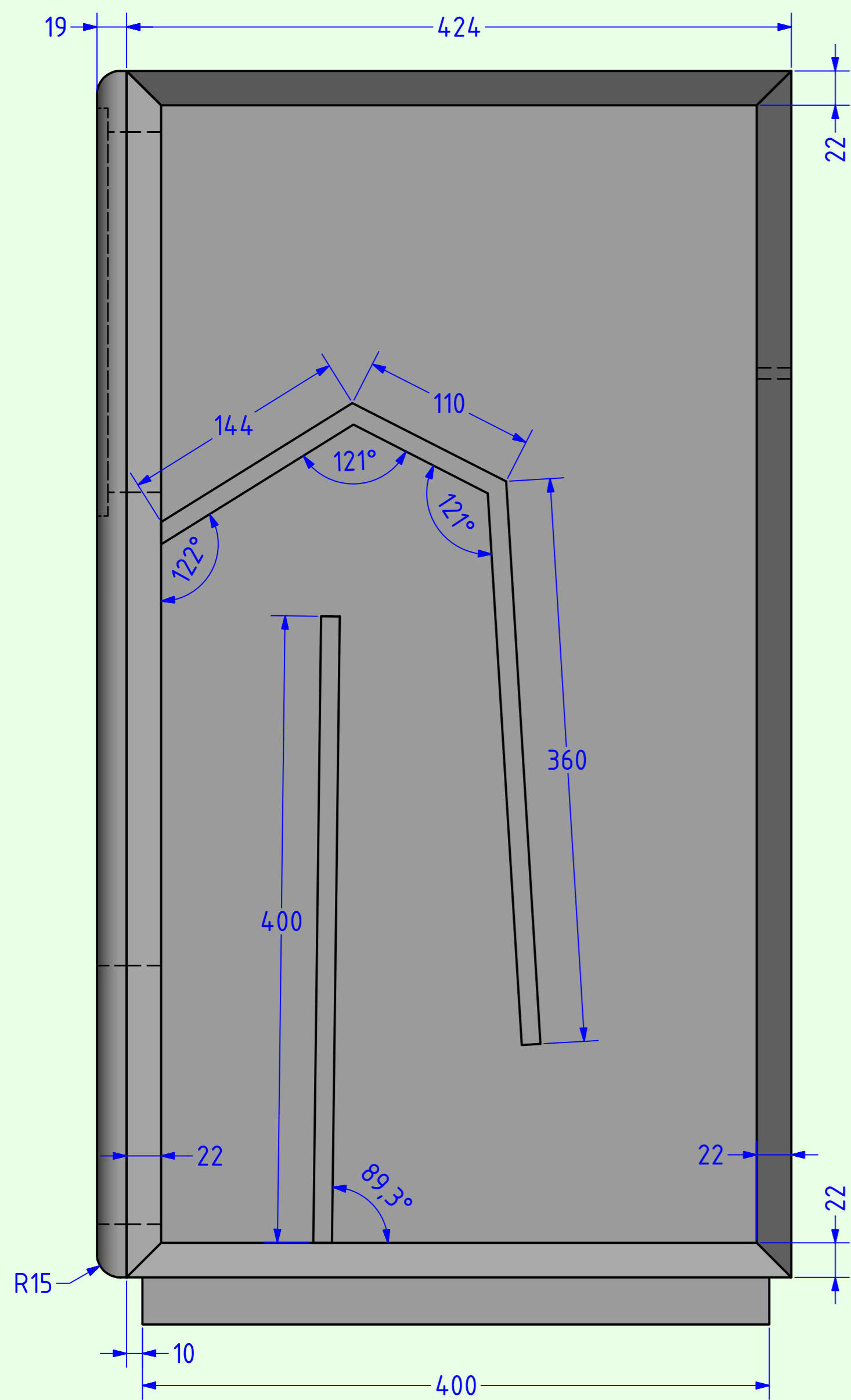
Seitenansicht (ohne rechte Seitenwand)
